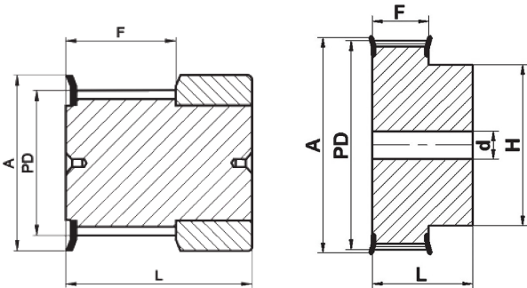
3М-06 AL Шаг зубьев: 3 mm Ширина ремня: 6 mm
