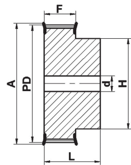
5M-09 ALШаг зубьев: 5 mm Ширина ремня: 9 mm
