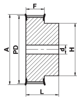
AT5-10 AL Шаг цепи: 5 mm Ширина ремня: 10 mm
