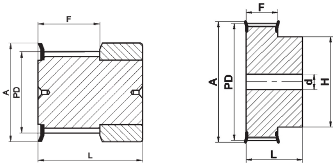
T2,5-06 ALШаг цепи: 2,5 mm Ширина ремня: 6 mm
