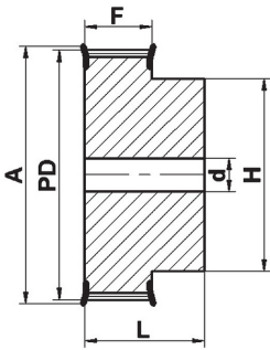
5M-09 Шаг цепи: 5 mm Ширина ремня: 9 mm
